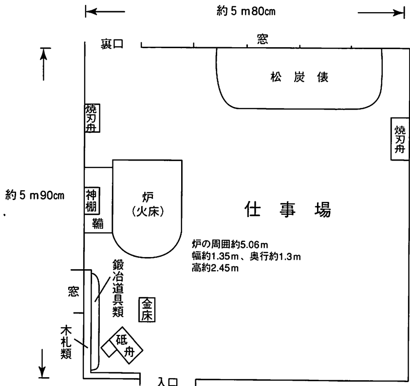
鍛錬場略図(平成13年調査)
